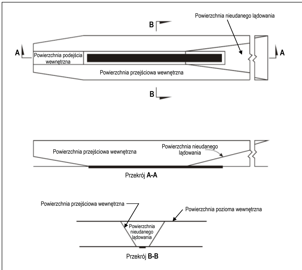
Rysunek 4-2. Powierzchnie ograniczające przeszkody: powierzchnia podejścia wewnętrzna, przejściowa wewnętrzna i nieudanego lądowania.
