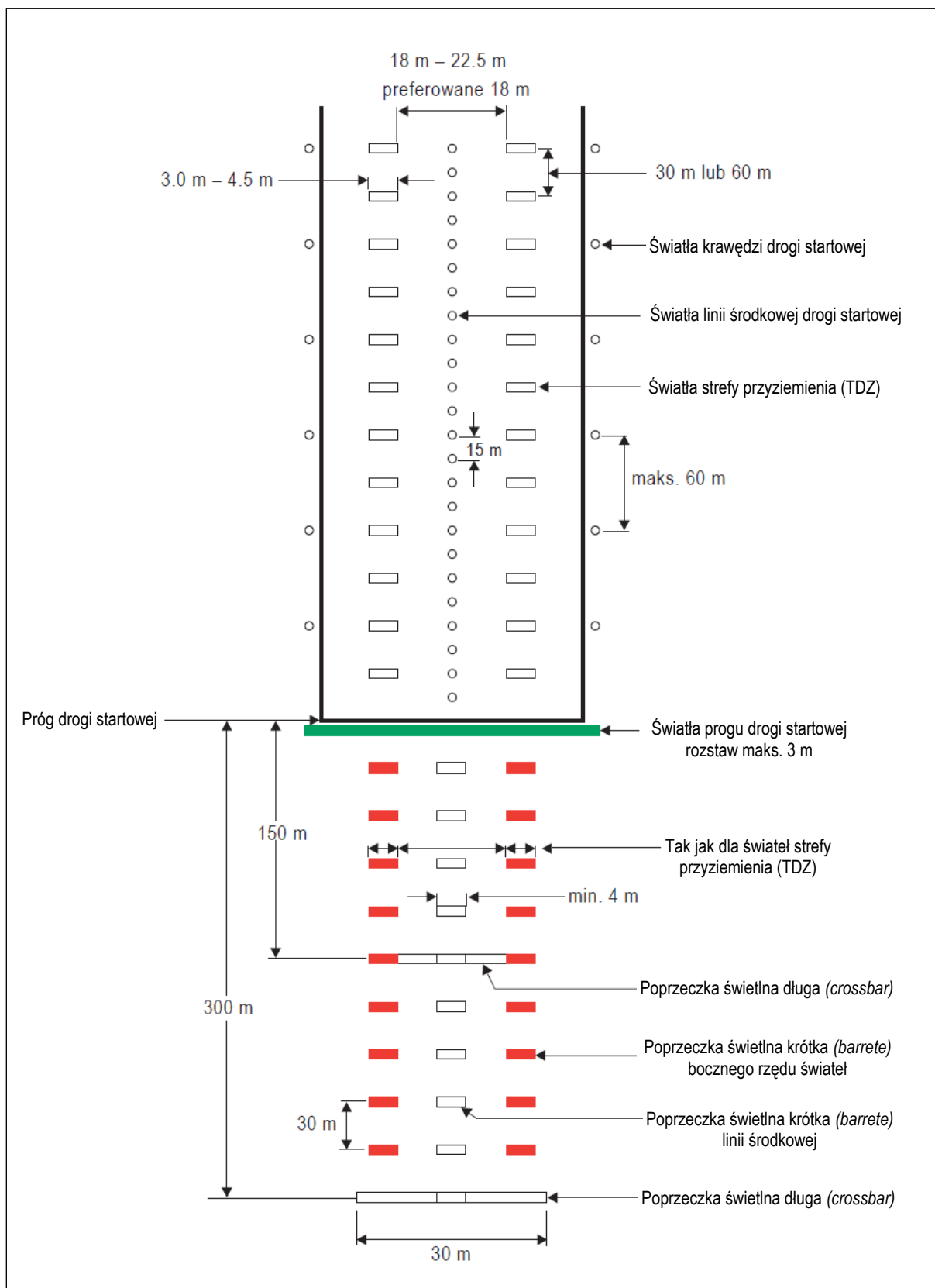
Rysunek 5-14. Wewnętrzny, 300 m odcinek podejścia oraz światła dla dróg startowych podejścia precyzyjnego kategorii II i III
