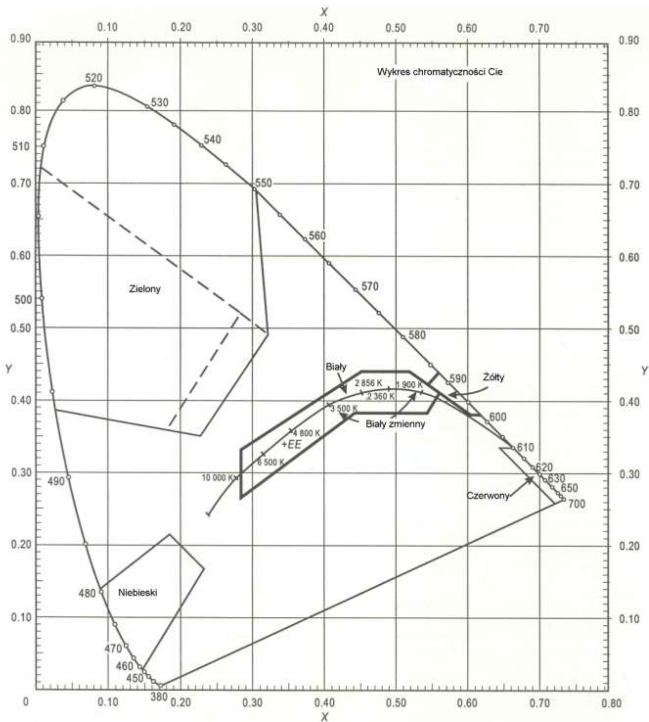
Rysunek D1-1. Kolory naziemnych świateł lotniczych
