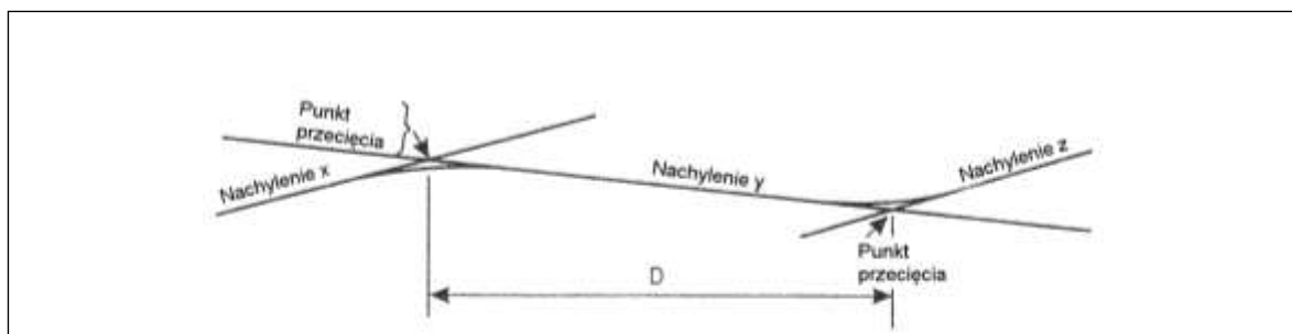
Rysunek ZA-2. Profil podłużny wzdłuż linii środkowej drogi startowej
