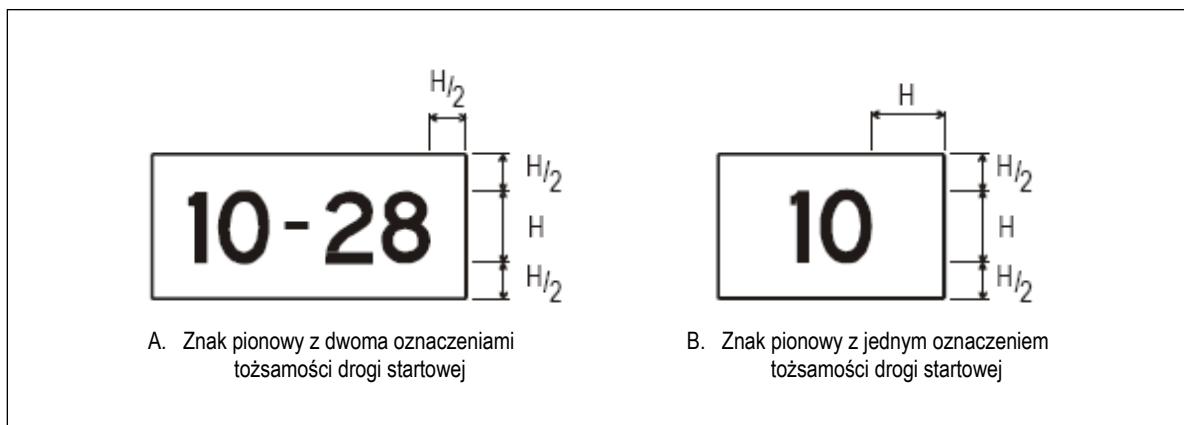
Rysunek D4-3. Wymiary znaku
