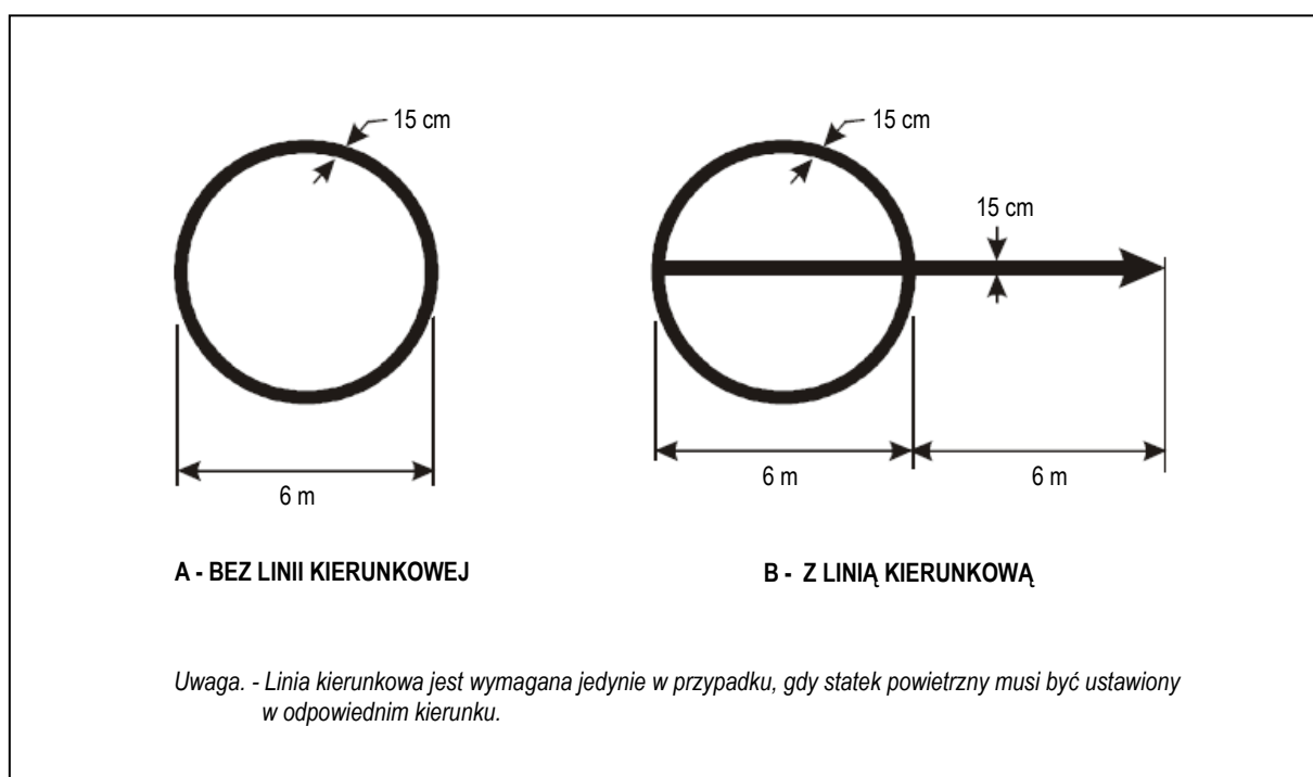
Rysunek 5-9. Oznakowanie poziome stanowiska sprawdzania VOR
