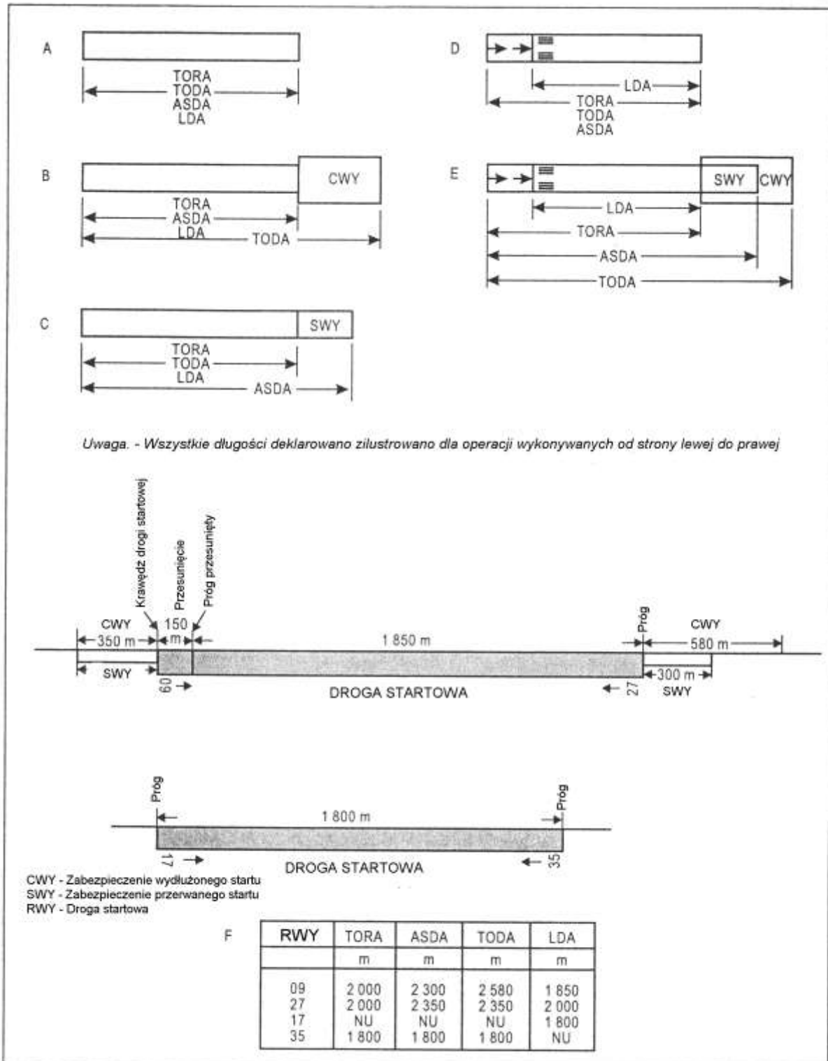
Rysunek ZA-1. Ilustracja długości deklarowanych
