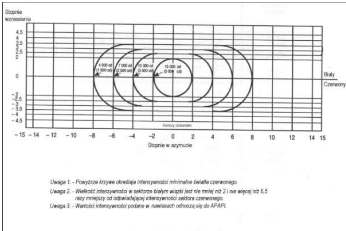
Rysunek D2-23. Rozkład intensywności światła PAPI oraz APAPI
