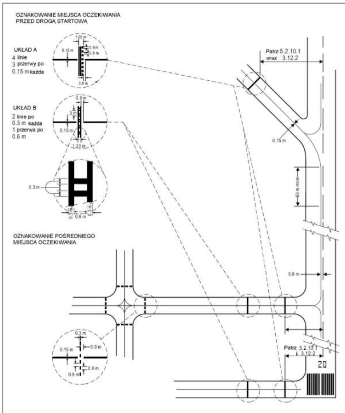
Rysunek 5-6. Oznakowanie drogi kołowania (przedstawione w połączeniu z podstawowymi znakami drogi startowej)
