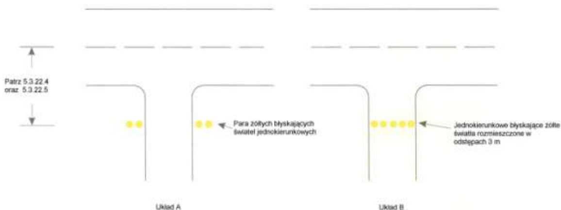
Rysunek 5-29. Światła ochronne drogi startowej
