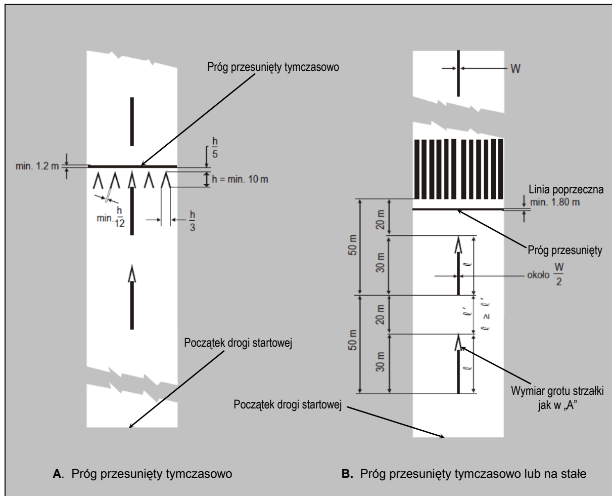
Rysunek 5-4. Oznakowanie przesuniętego progu
