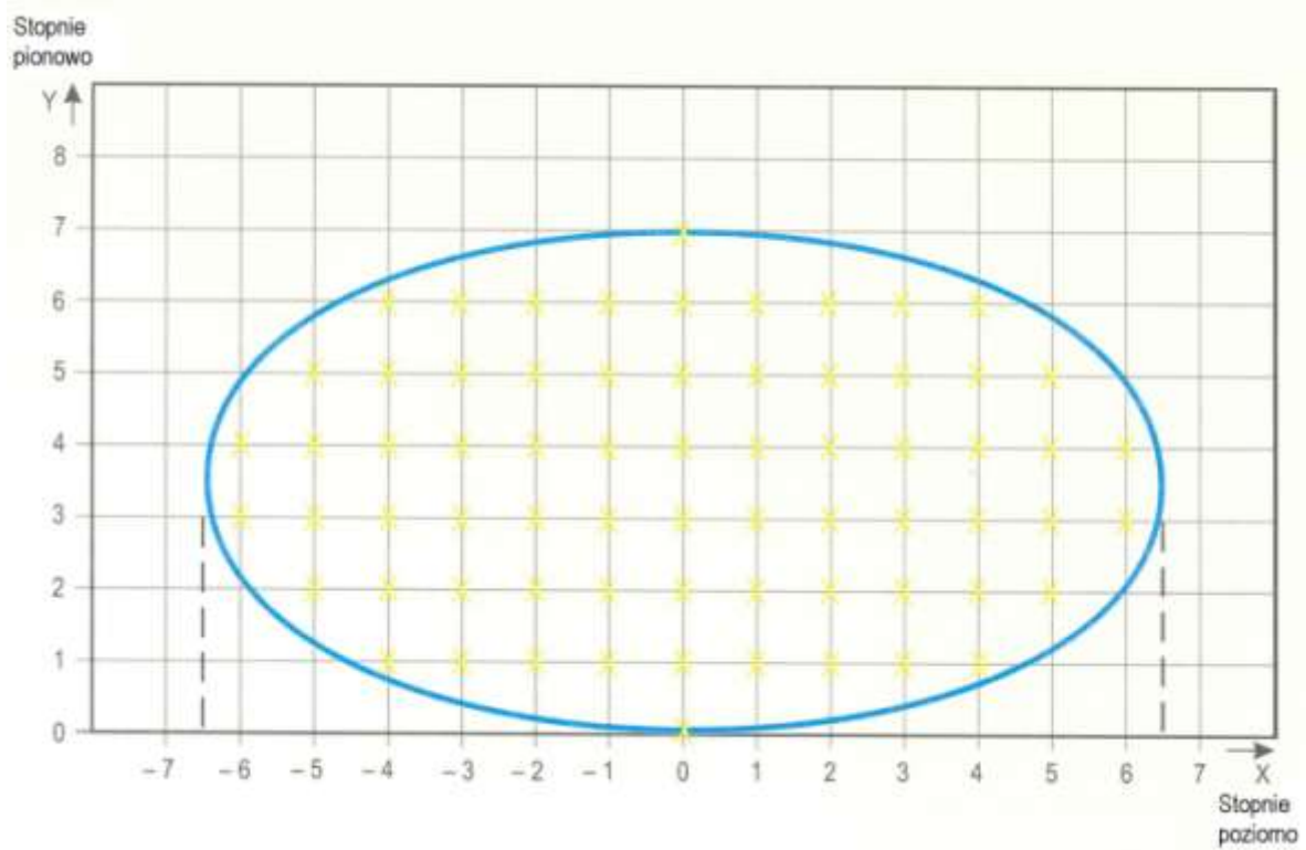
Rysunek D2-11. Punkty siatki służące do obliczeń średniej intensywności świateł systemu podejścia oraz drogi startowej
