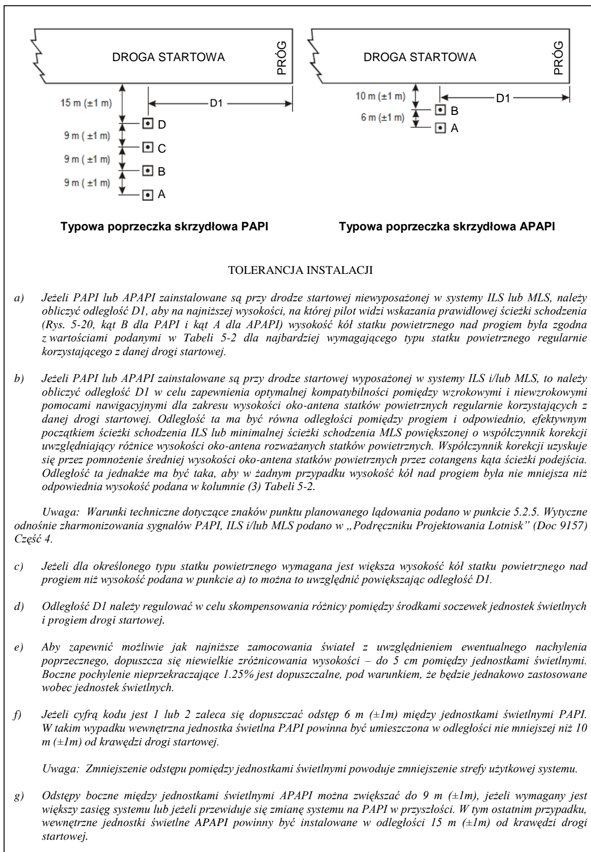
Rysunek 5-19. Ustawienie PAPI i APAPI
