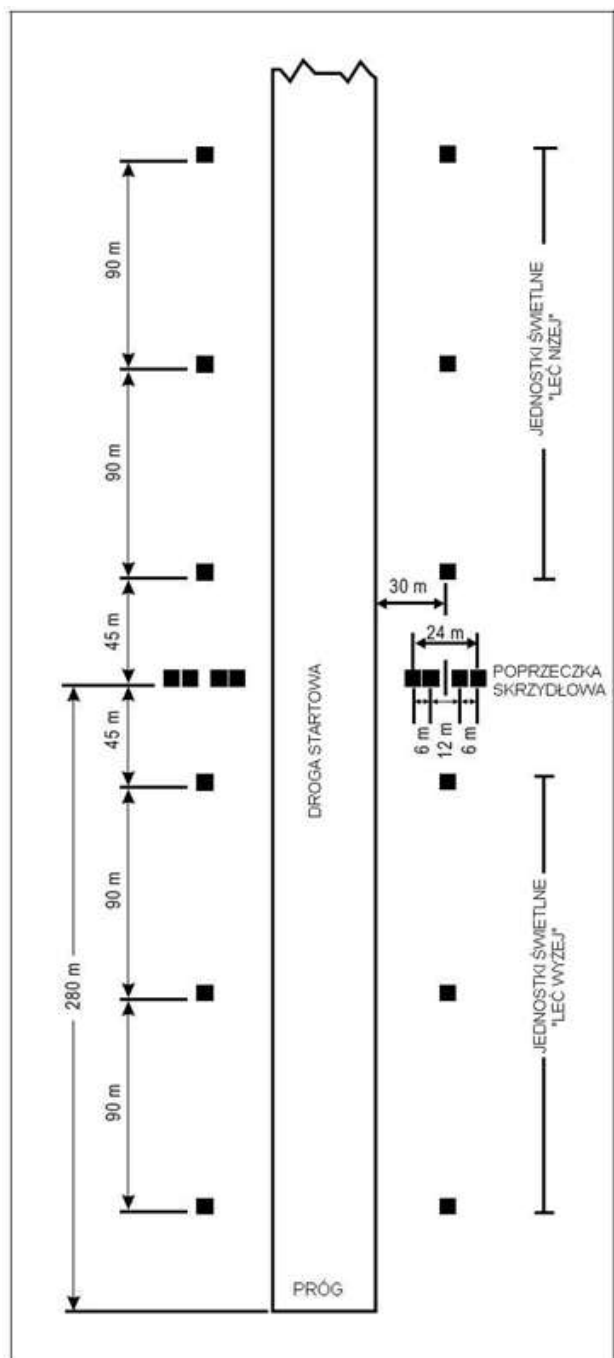
Rysunek 5-17. Rozmieszczenie jednostek świetlnych systemu T-VASIS
