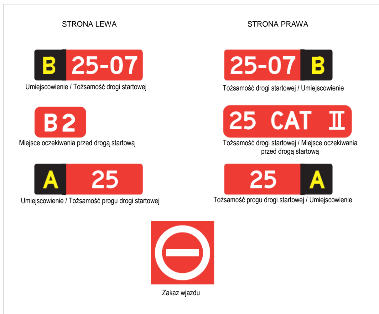
Rysunek 5-30. Pionowe znaki nakazu
