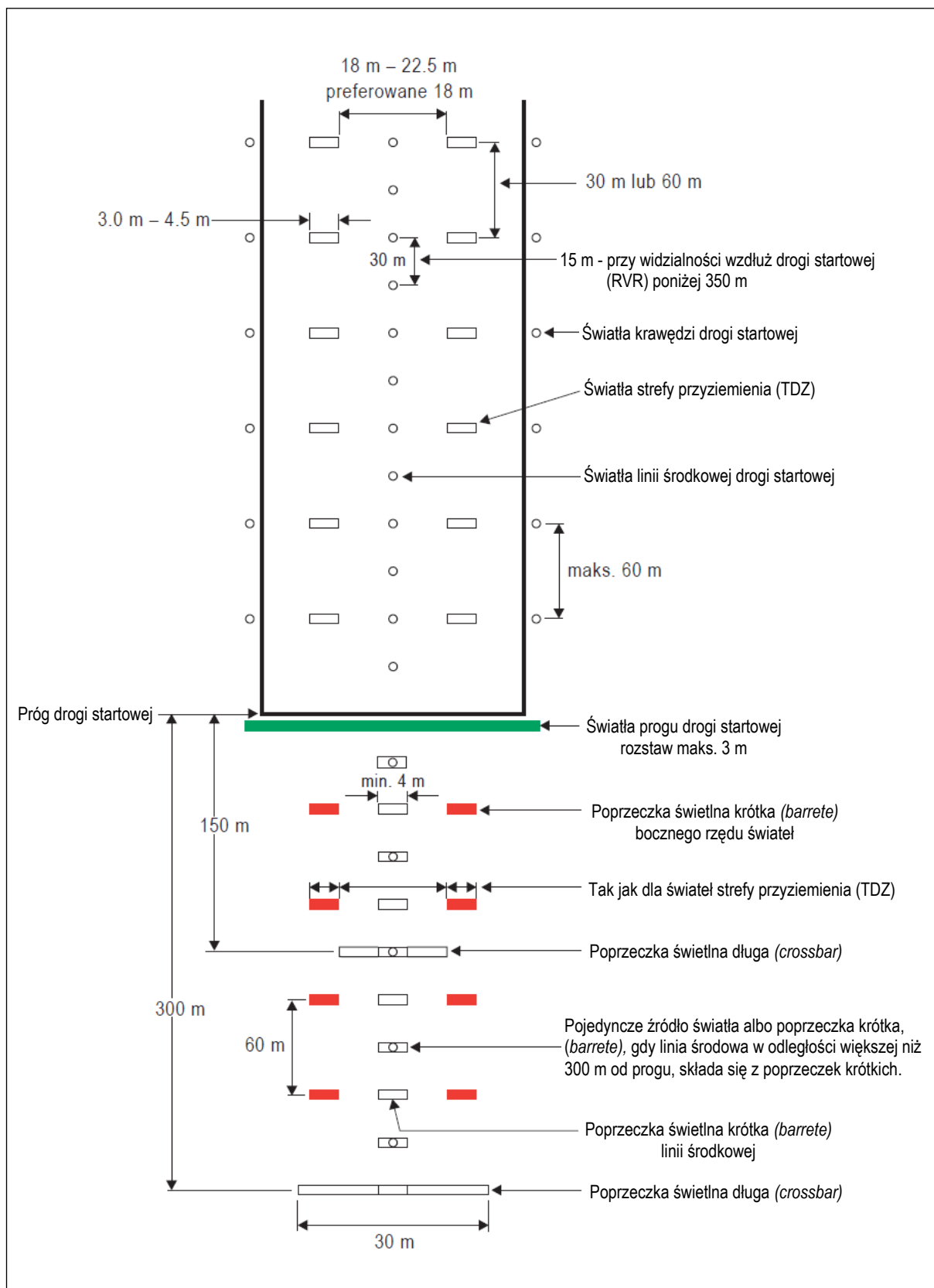
Rysunek 5-15 Wewnętrzny, 300 metrowy odcinek podejścia oraz światła dla dróg startowych z podejściem precyzyjnym kategorii II i III, dla których mogą być zapewnione, jako warunek eksploatacji, poziomy niezawodności świateł określone w Rozdziale 10
