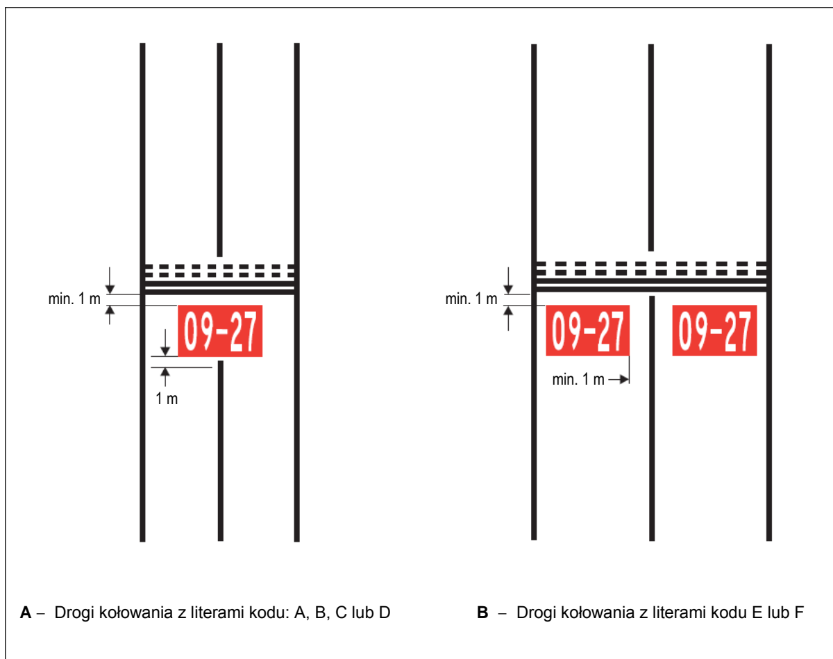
Rysunek 5-10. Oznakowanie nakazu
