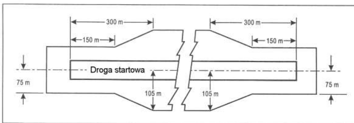
Rysunek ZA-4. Wyrównana część pasa drogi startowej o cyfrze kodu 3 lub 4 z podejściem precyzyjnym
