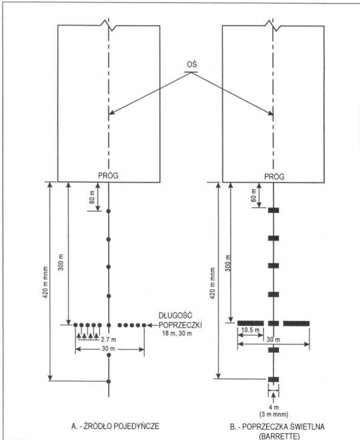
Rysunek A-7. Uprozczone świetlne systemy podejścia
