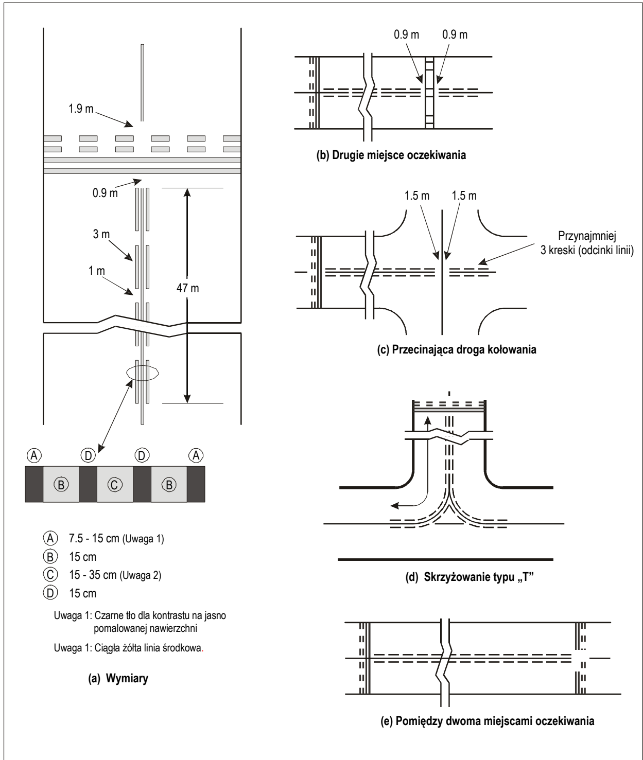
Rysunek 5-7. Bardziej wyraziste oznakowanie linii środkowej drogi kołowania
