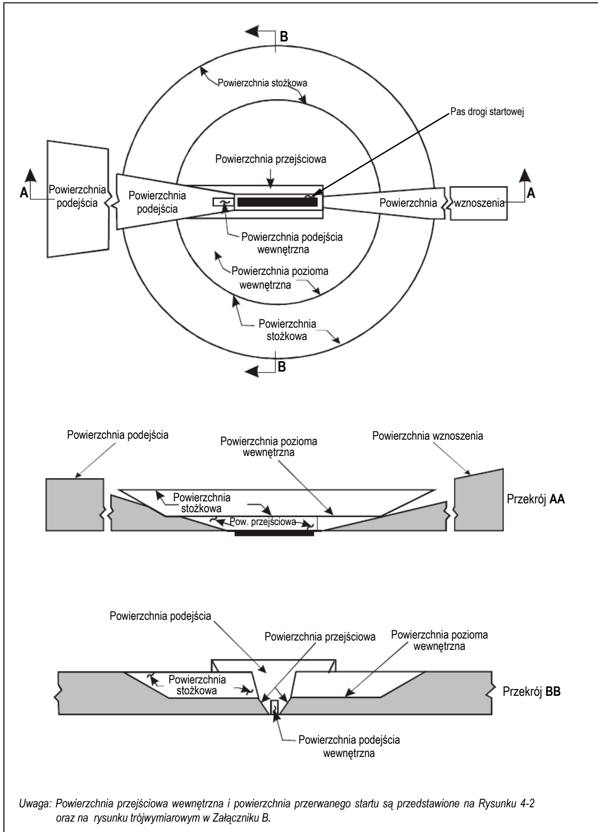
Rysunek 4-1. Powierzchnie ograniczające przeszkody.
