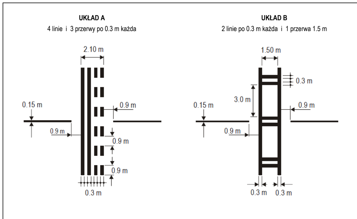
Rysunek 5-8. Oznakowanie poziome miejsca oczekiwania przed drogą startową
