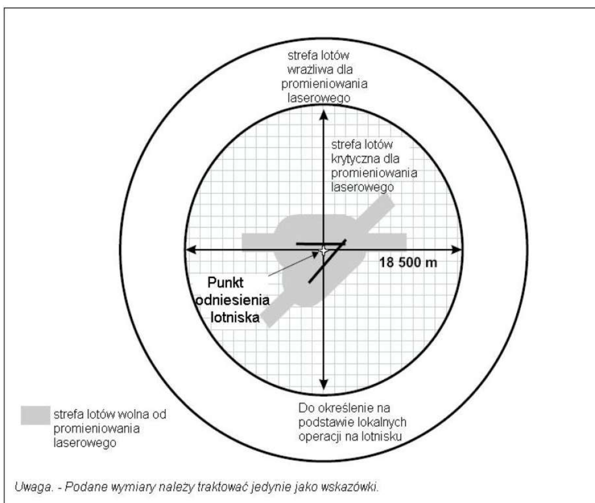
Rysunek 5–11. Strefy ochronne lotów
