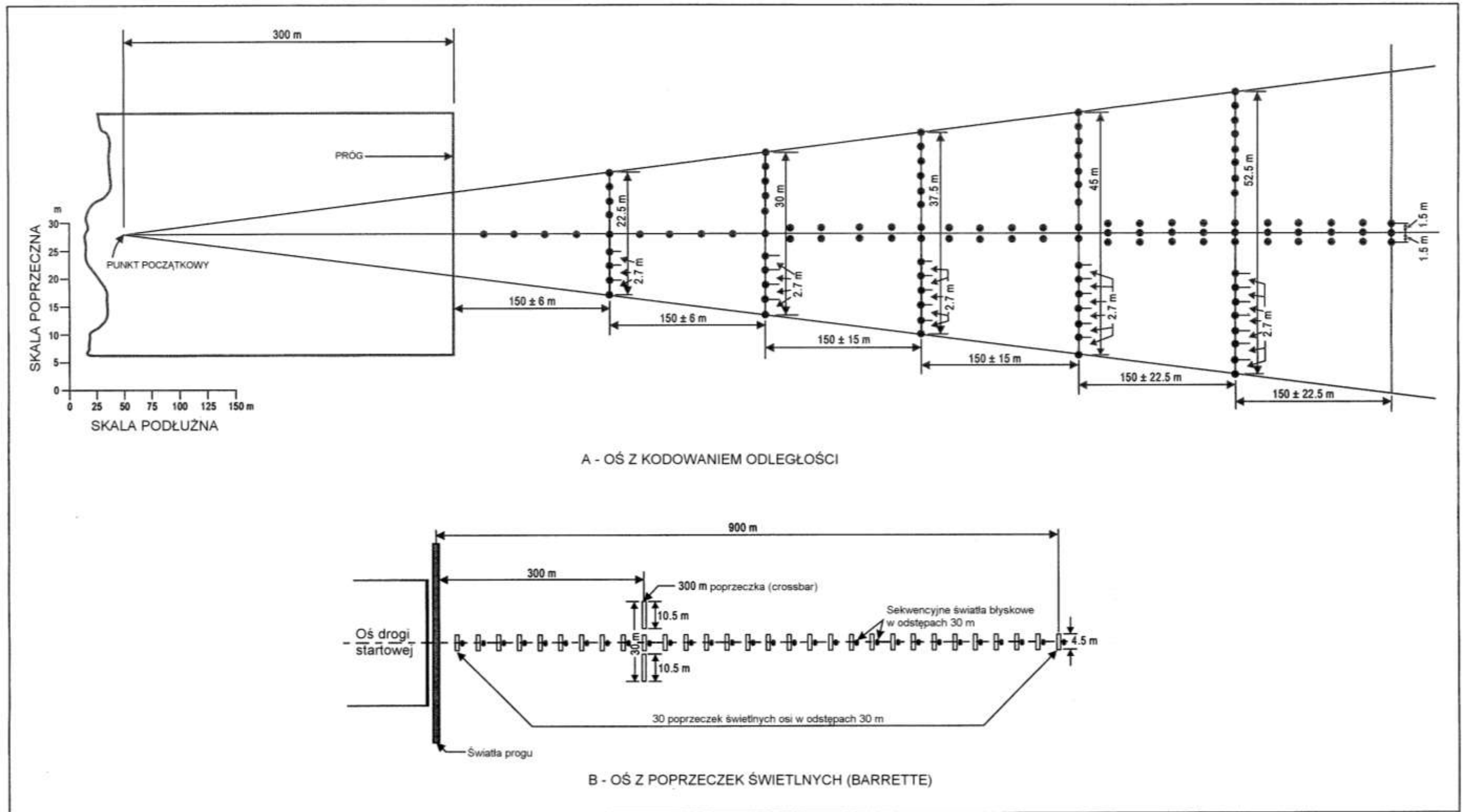
Rysunek A-8. Światłne systemy podejścia precyzyjnego kategorii I
