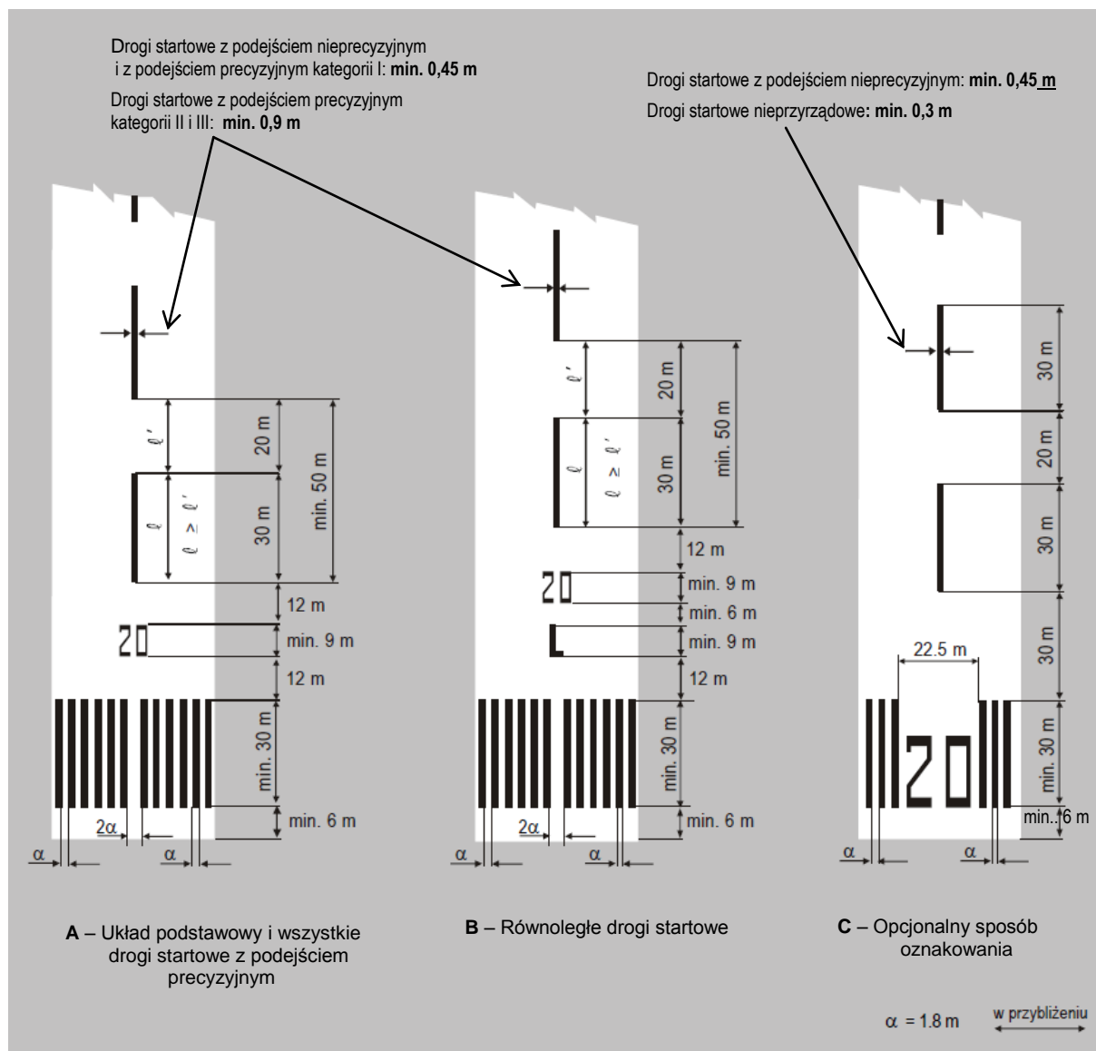
Rysunek 5-2. Oznakowanie linii środkowej, progu oraz identyfikacji drogi startowej
