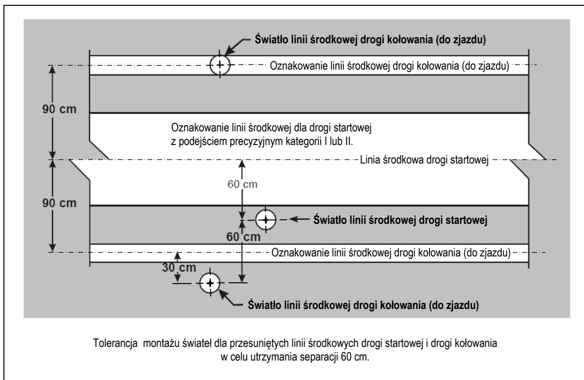
Rysunek 5-27. Światła przesuniętej linii środkowej drogi startowej i linii środkowej drogi kołowania
