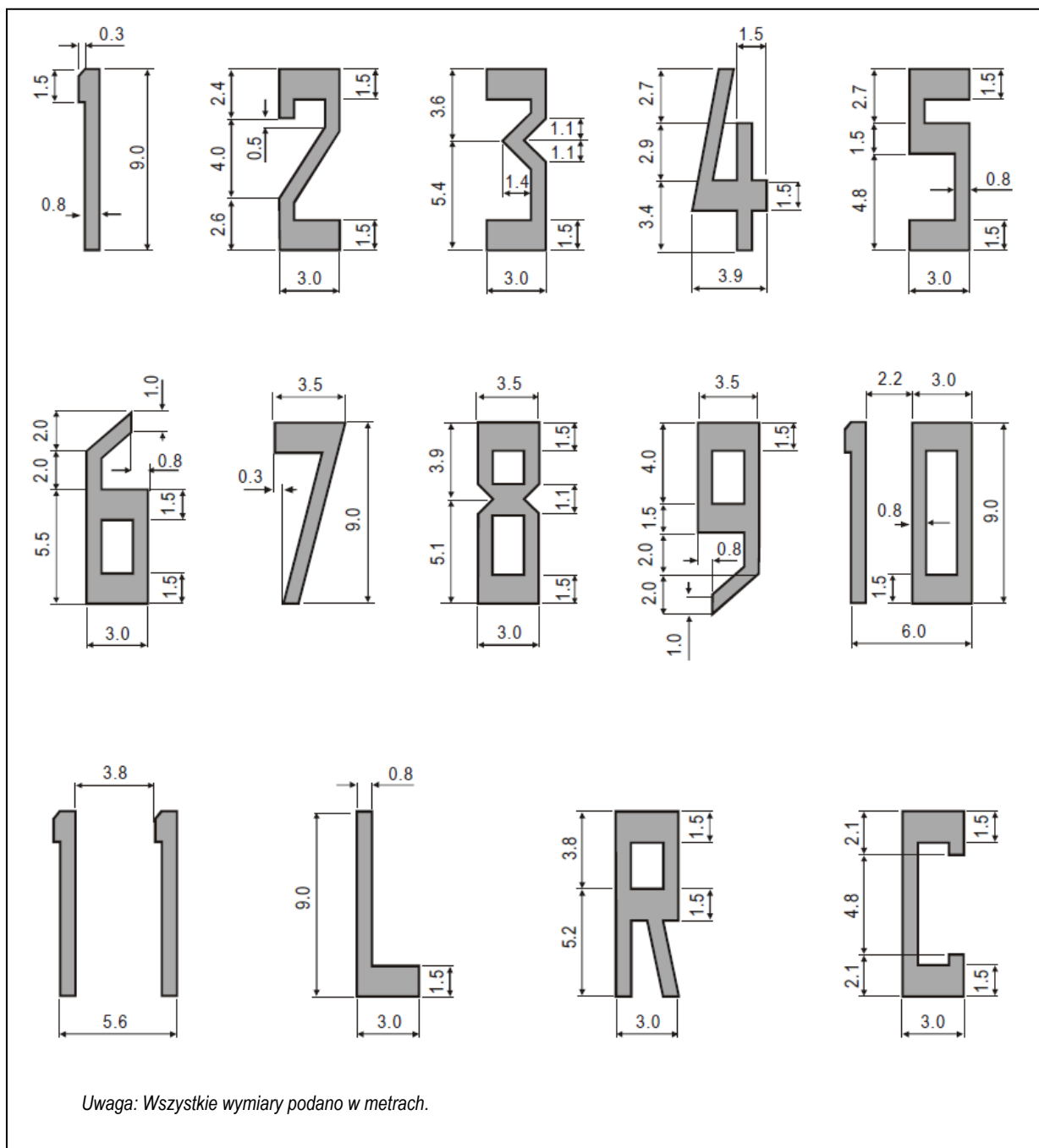
Rysunek 5-3. Kształt i proporcje liter i cyfr używanych do oznakowania identyfikacji drogi startowej
