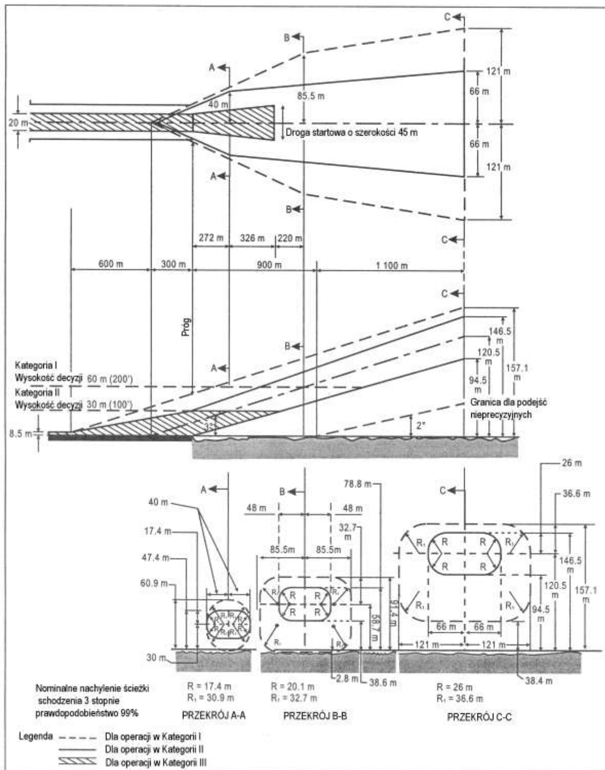
Rysunek A-6. Obwiednie trajektorii lotu używane do projektowanie świateł dla operacji w warunkach I, II oraz III kategorii
